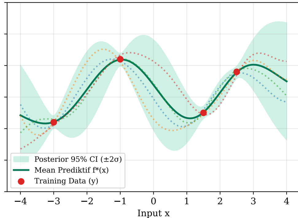
(b) Posterior Gaussian Process (Setelah Observasi)
